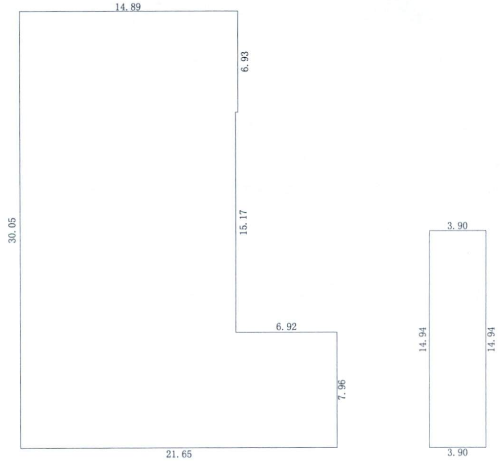
四层平面图
