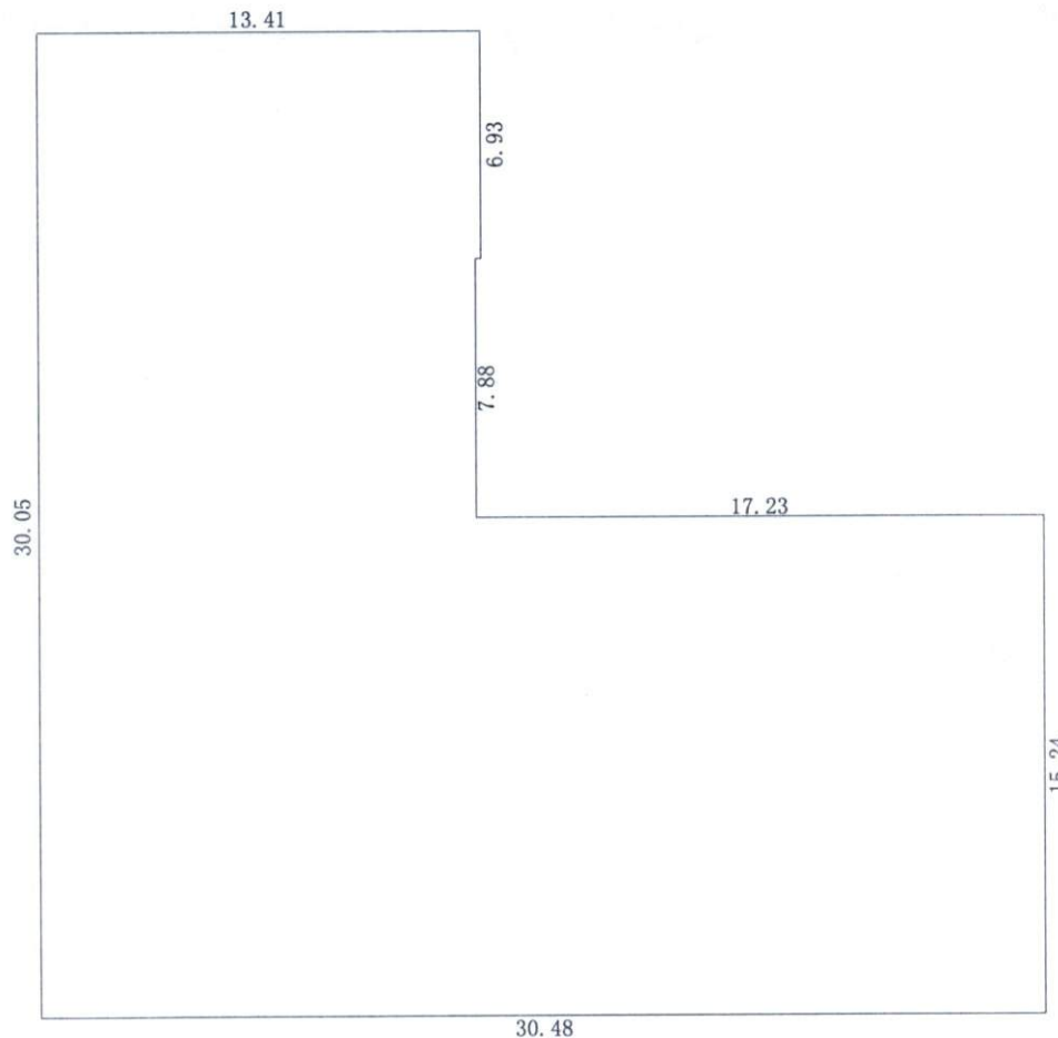
二层平面图
