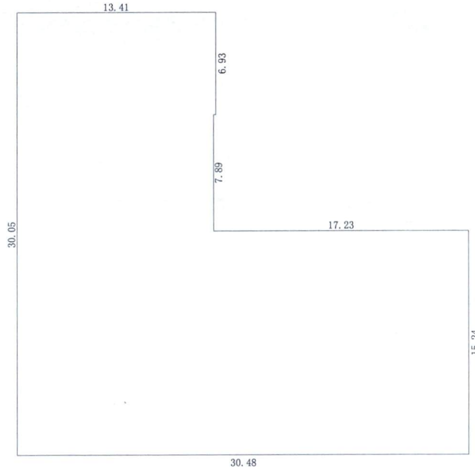
一层平面图
